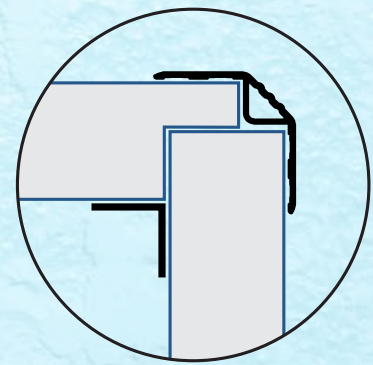
Kältebrückenfreie Konstruktion
